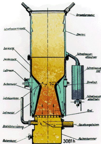
Bild 8. Kromag-Holzgasleingenerator Type „K“
