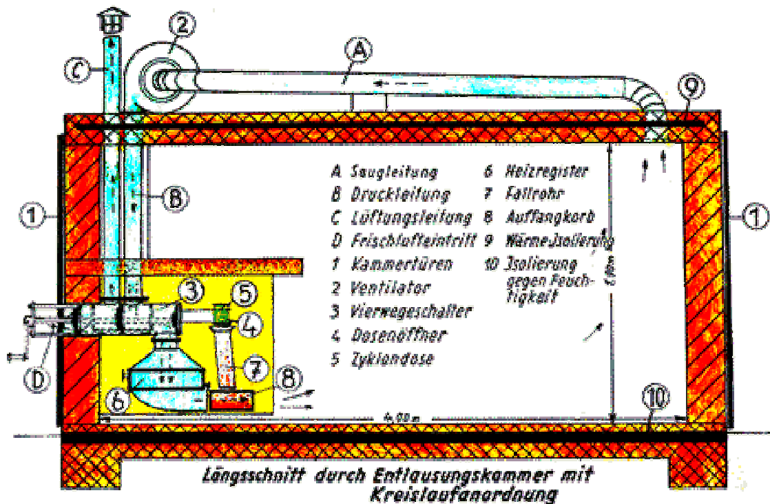
Abb. 26. Längsschnitt durch eine Entlausungskammer mit Kreislaufanordnung
