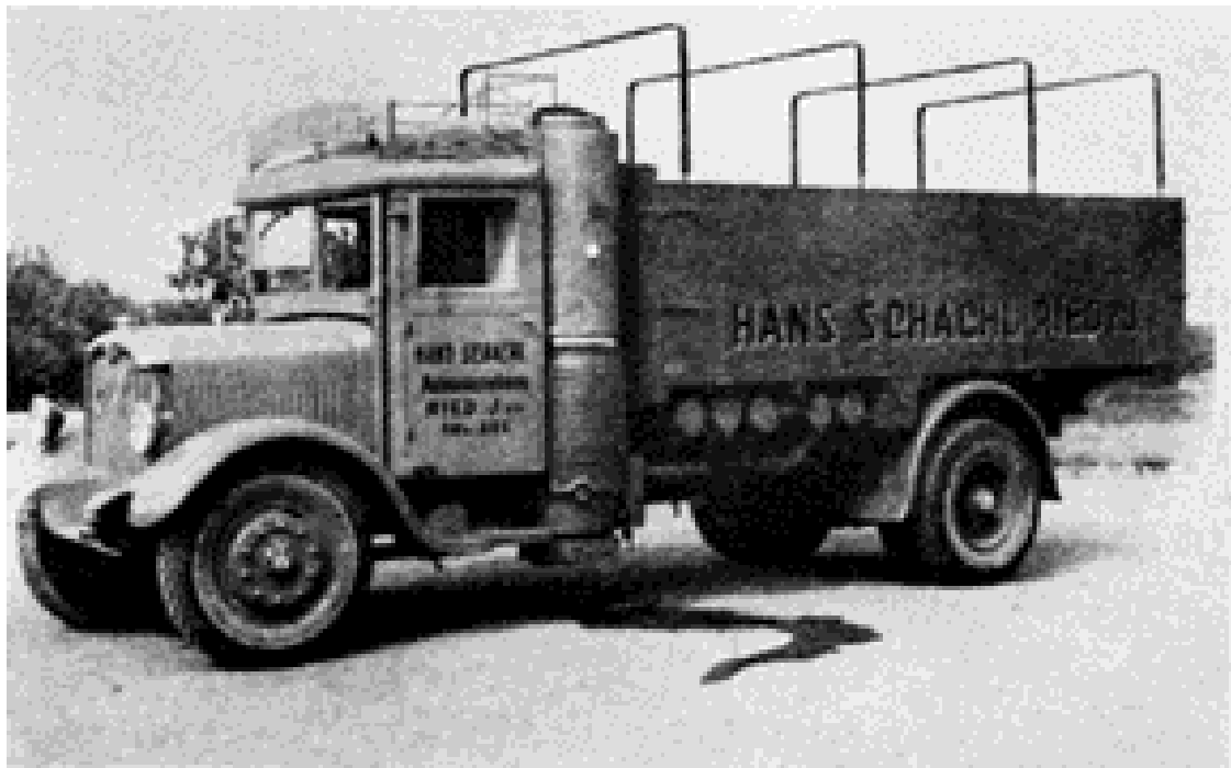
Abb. 1. Saurer 5 BHW. mit Holzgasantrieb.
